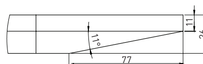
Sloping edge
